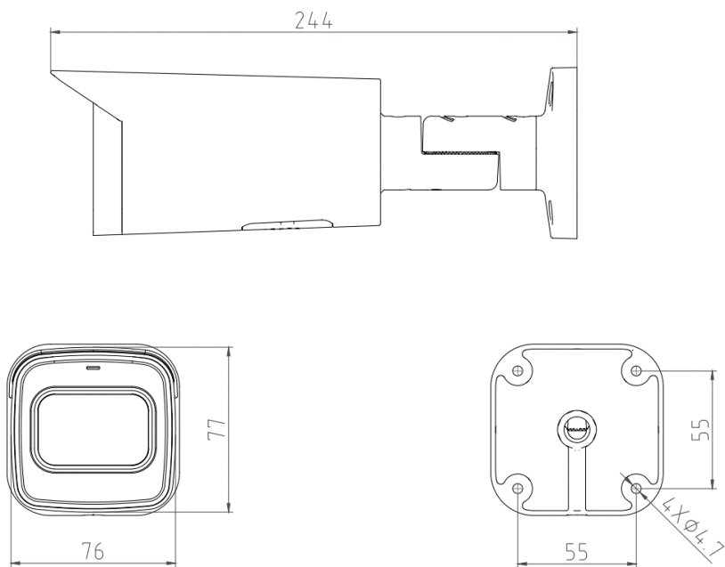
Габаритные размеры
