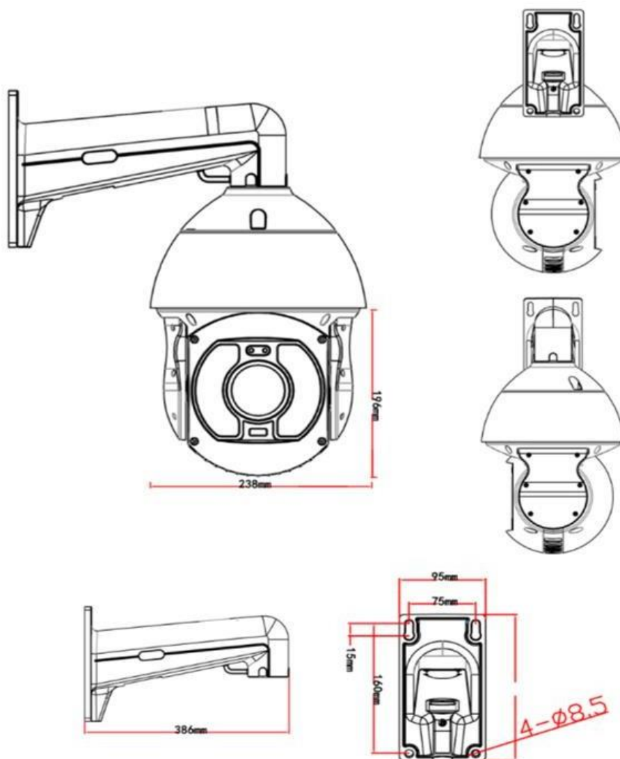
Габаритные размеры в мм
